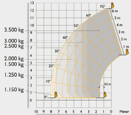
535-125 mit ausgefahrenen HiViz-Stabilisatoren
